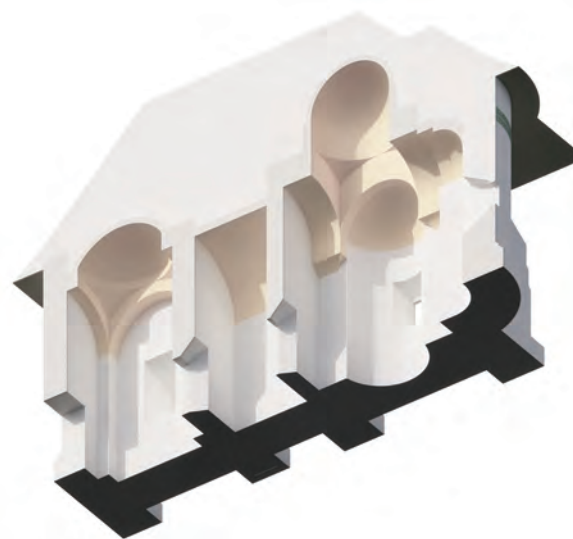
Figura 7. Reconstituirea arhitecturală a bisericii Mănăstirii Bistrița, varianta 1: a. Plan și secțiune; b. Reconstituire 3D (Alma Vasile).
