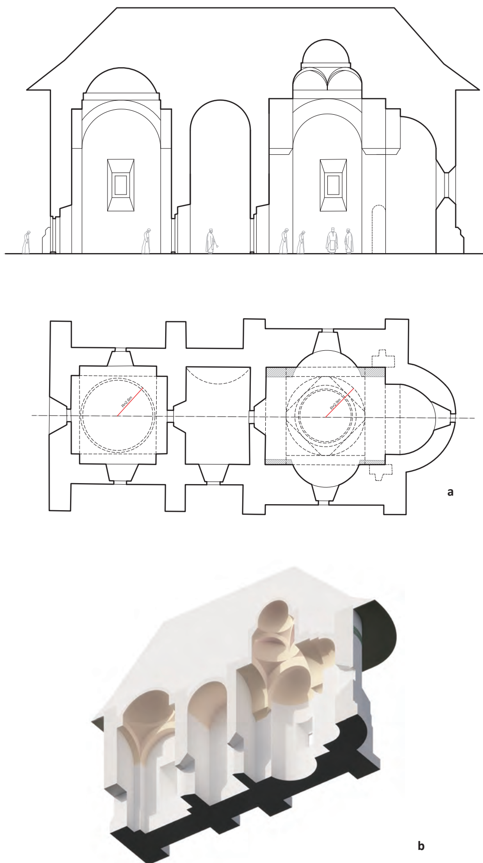
Figura 8. Reconstituirea arhitecturală a bisericii Mănăstirii Bistrița, varianta 2: a. Plan și secțiune; b. Reconstituire 3D (Alma Vasile). Figure 8. Architectural reconstruction of Bistrița Monastery Church, version 2: a. Plan and section; b. 3D reconstruction (Alma Vasile).
